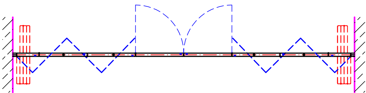
Mittelpunkt Aufhängung Zweiflügelig mit Stand – und Gehflügel
